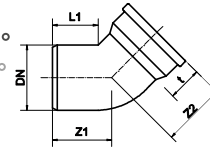
Bogen 15° - 88° Bends 15° - 88°
